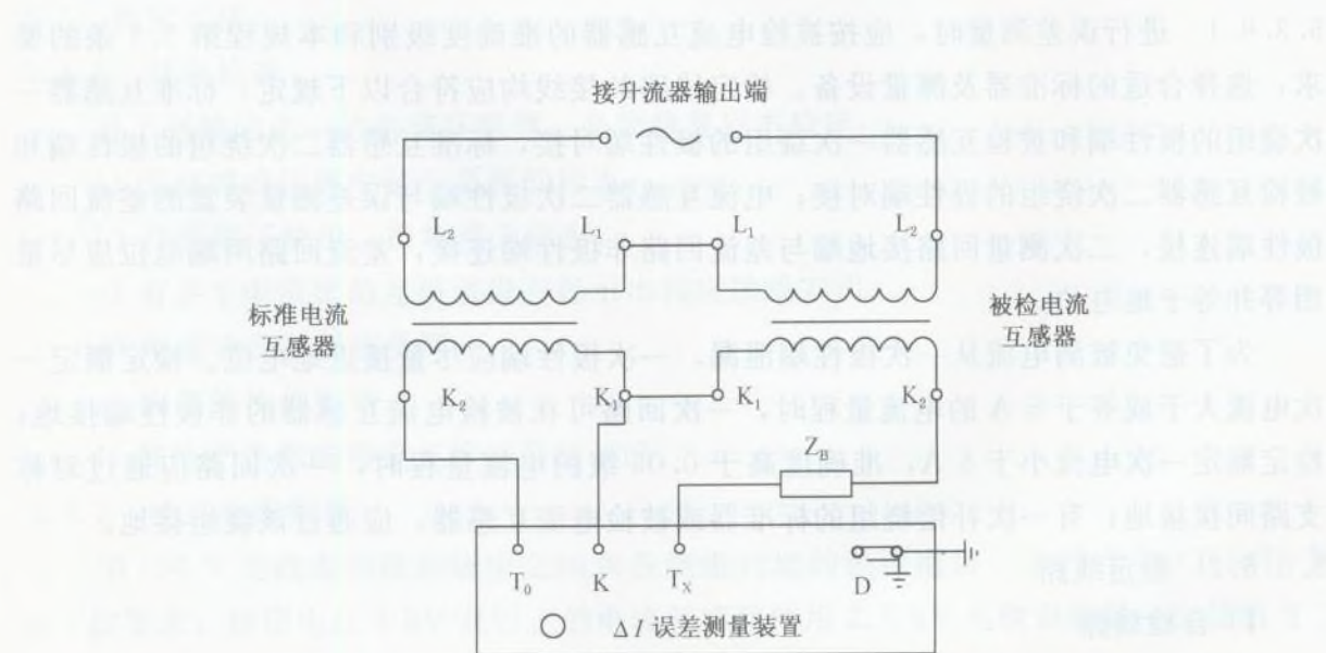
图 1 电流互感器自检线路
