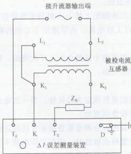
图 1 电流互感器自检线路
