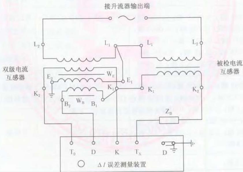
图8 一次补偿绕组接地线路
