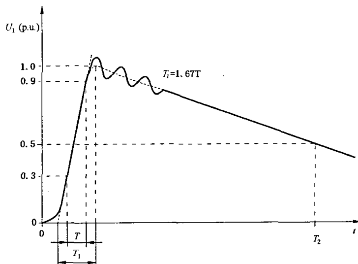
A类波形
