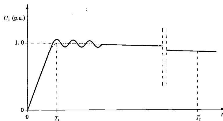
B类波形
