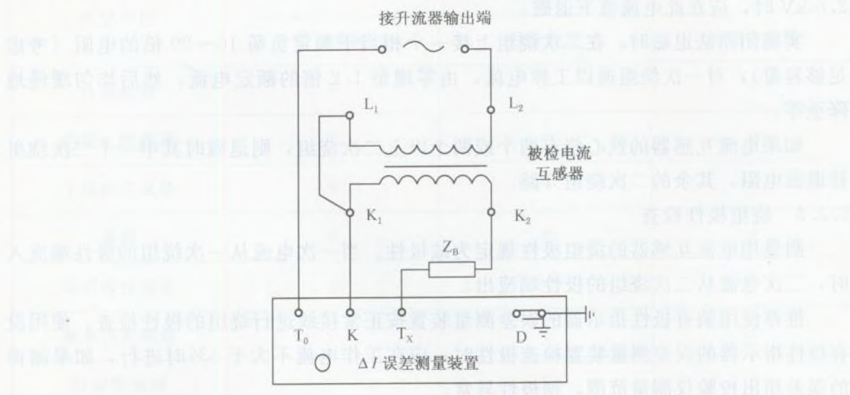
图 1 电流互感器自检线路
