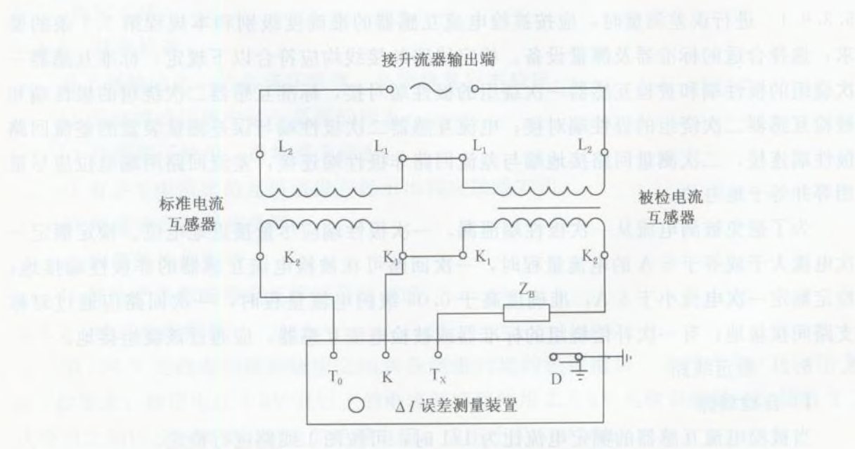
图 2 电流互感器比较法检定线路
